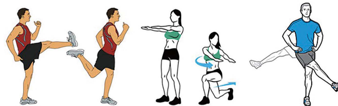
Gambar 2. Peregangan dinamis
