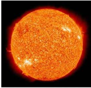
Gambar 16.3. Matahari: bola gas raksasa yang sangat besar Sumber: id.wikipedia.org
