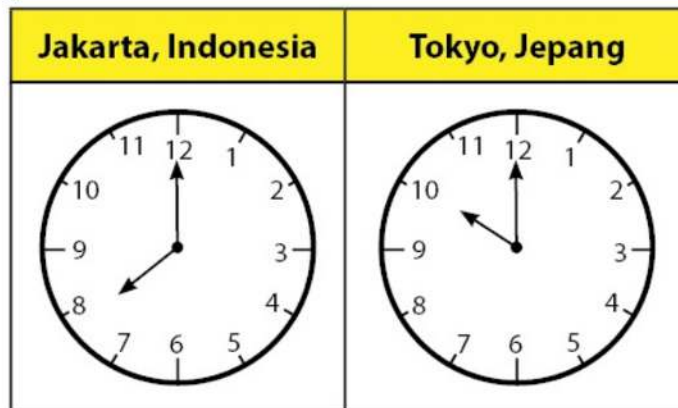
Gambar 16.21. perbedaan waktu Sumber: idschool.net
