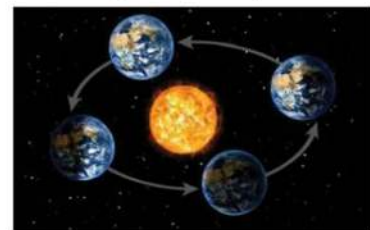
Gambar 16.22. Proses Rotasi Bumi
