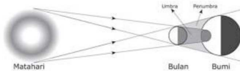
Gambar 16.28. Terjadinya Gerhana Matahari
