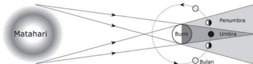
Gambar 16.27. Gerhana Bulan Total dan Sebagian
