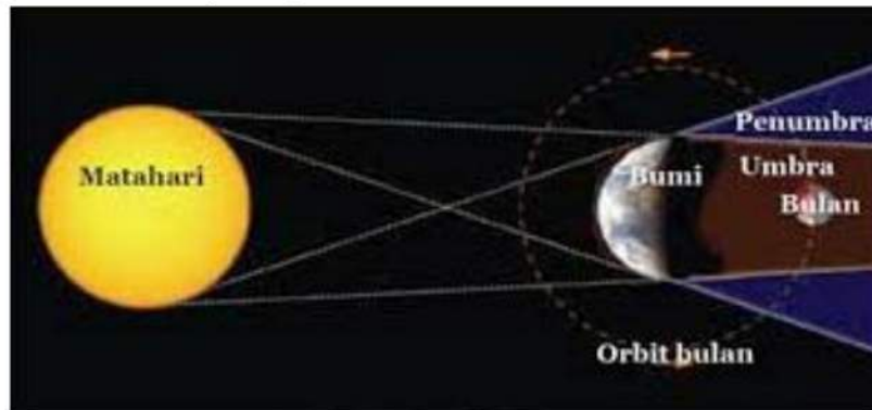
Gambar 16.25. Gerhana Bulan Sumber: pelajarankelasku.blogspot
