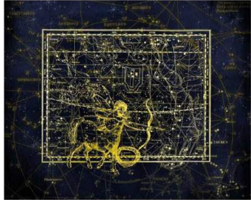
Gambar 16.23. perubahan rasi bintang
