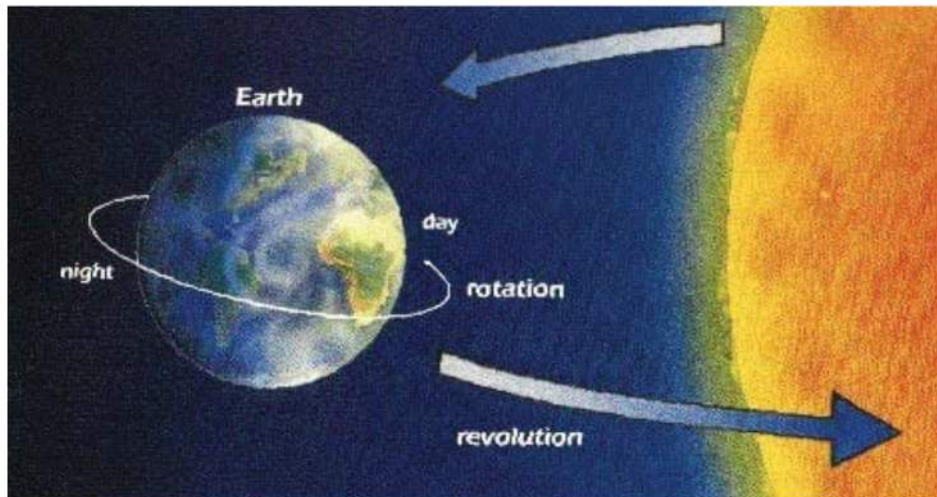
Gambar 16.18. Alur Rotasi dan Revolusi Bumi Sumber : duniapendidikan.co.id
